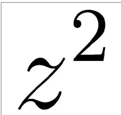
Abb. 2: PostScript-Font.
