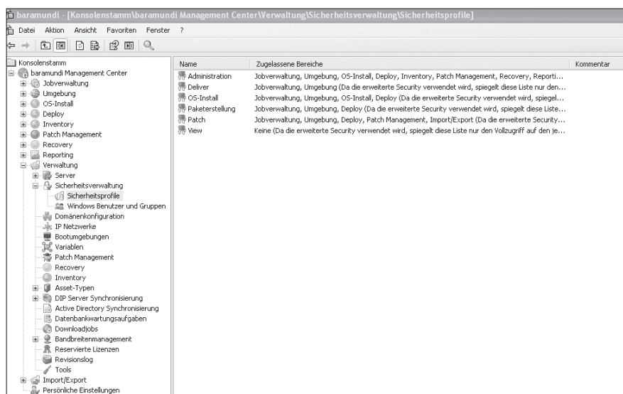
Abb. 2: Baramundi Oberfläche
