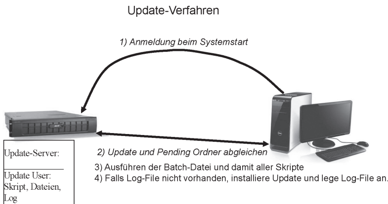
Abb. 1: Update-Verfahren
