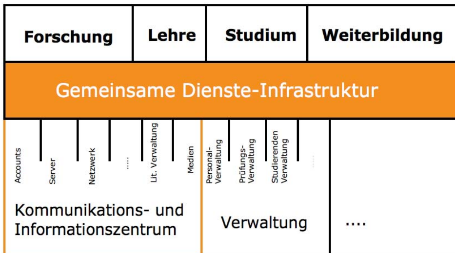
Abbildung 2: Gemeinsame Dienstinfrastruktur
