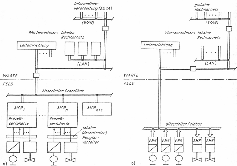
Abbildung 2: Lokale Rechnernetze LAN in Automatisierungsanlagen a) Industriestruktur TDC 3000, Fa. Honeywell, seit 1983; b) Systemstruktur mit Feldbus und Einchip-Mikrorechnern EMR in den Geräten: intelligente, direkt buskopplbare Mess- und Stellgeräte sowie Leiteinrichtungen mit Kopplung an LAN und WAN [27]
