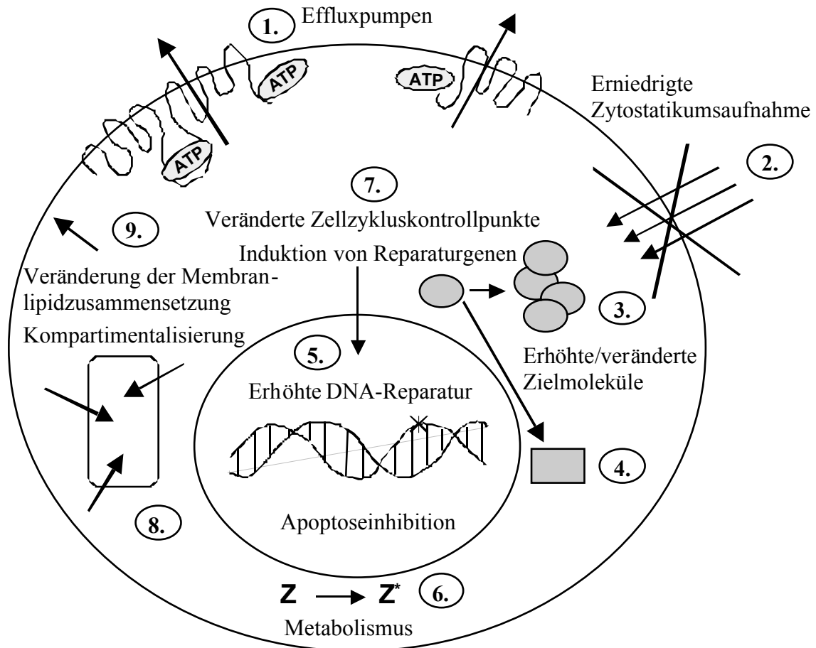
Abbildung 3: Mechanismen der Chemoresistenz (verändert nach Gottesman, 2002)
