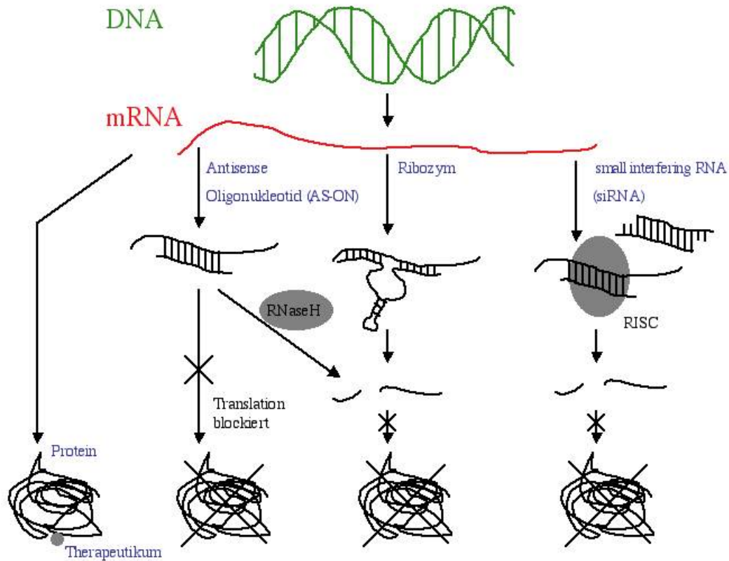
Abbildung 4: RNA-Technologien zur Geninhibition (verändert nach: Kurreck, 2003)
