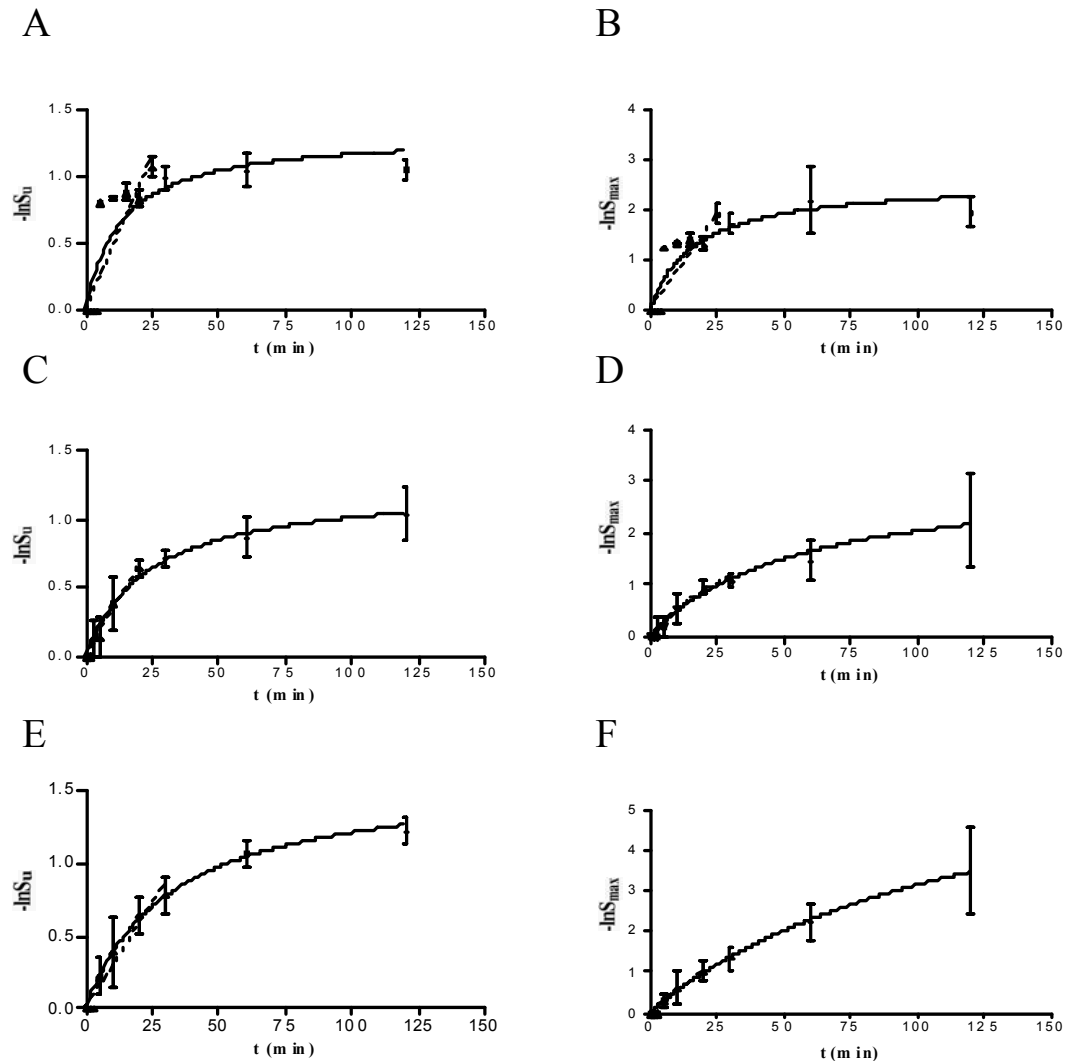
Abbildung 16: Der Reaktionsparameter k_{\text{obs}} für die Katalyse der Substrat-RNAs
