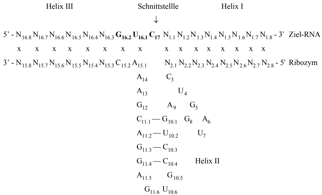
Abbildung 5: Struktur eines Hammerhead -Ribozymes
