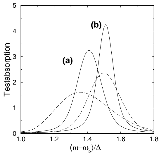
Abbildung 4.26: Verschobene Testabsorption für unterschiedliche Zerfallsraten der Pump photons \gamma_c . (a): \gamma_c = 0,25g , \kappa = 0,1g , \langle b^\dagger b \rangle = 50 ; (b): \gamma_c = g , \kappa = 0,2g , \langle b^\dagger b \rangle = 200 . Durchgezogene Kurven: \xi = 0 , gestrichelte Kurven: \xi = -1 . Weitere Parameter: N = 1 , \Delta = 10g , \Delta_c = 0 , \gamma_r = 0,5g .
