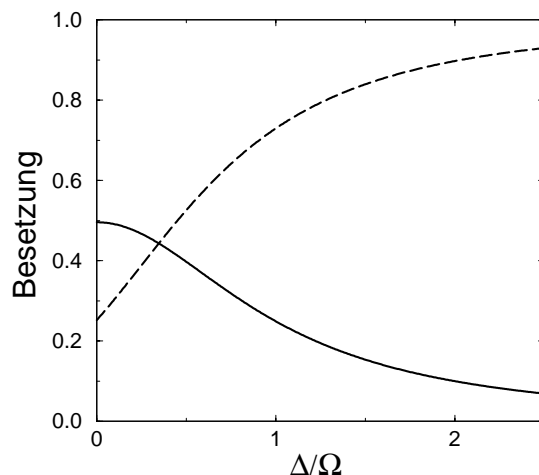
Abbildung 2.13: Besetzung der 'Dressed States' innerhalb des Triplets mit n = 60 für zwei TLS ( N = 2 ) in Abhängigkeit von \Delta . Gestrichelte Kurve: Besetzung des unteren 'Dressed State'; durchgezogene Kurve: Besetzung des mittleren 'Dressed State'.
