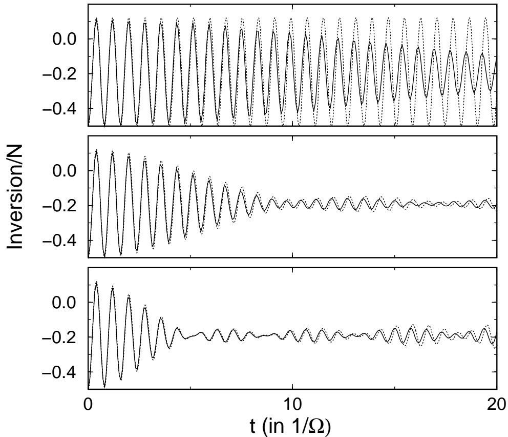
Abbildung 4.1: Zeitentwicklung der Inversion für unterschiedliche inhomogene Verteilungen. Oberes Bild: \Gamma = 0, 1g ; mittleres Bild: \Gamma = 2g ; unteres Bild: \Gamma = 4g . Das Pumpfeld ist in einem Fockzustand mit n = 60 Photonen. Parameter: N = 7 , \Delta = 12g . Durchgezogene Kurven: exakt; gepunktete Kurven: DMN.
