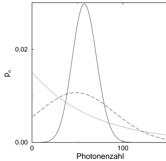
Abbildung 2.9: Photonenzahlverteilung der Laseremission für unterschiedliche Pumpparameter. Durchgezogene Kurve: r = 1,5 ; gestrichelte Kurve: r = 1,03 ; gepunktete Kurve: r = 0,98 ; mittlere Photonenzahl: \langle n \rangle = 100 .
