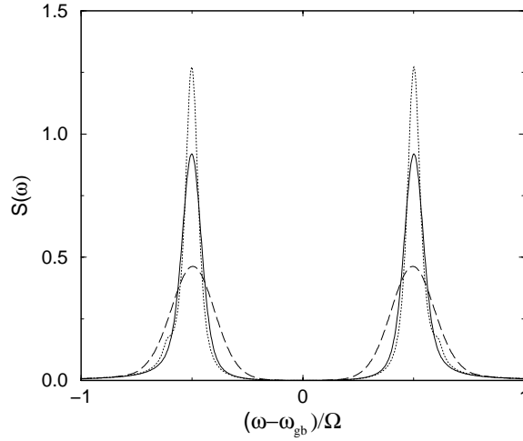
Abbildung 2.23: Autler-Townes-Spektrum für \langle n \rangle = 60 , \gamma = 0, 4g für unterschiedlich gequetschte Pumpfelder. Gepunktete Kurve: \xi = 1 ; gestrichelte Kurve: \xi = -1 ; durchgezogene Kurve: \xi = 0 .
