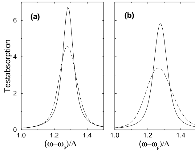
Abbildung 4.25: Verschobene Testabsorption für unterschiedliche Zerfallsraten der Pump photons \gamma_c . (a): \gamma_c = 3g , \kappa = 0 , \langle b^\dagger b \rangle = 290 ; (b): \gamma_c = g , \kappa = 0 , \langle b^\dagger b \rangle = 100 . Durchgezogene Kurven: \xi = 0 , gestrichelte Kurven: \xi = -1 . Weitere Parameter: N = 1 , \Delta = 10g , \Delta_c = 0 , \gamma_r = 0,5g .
