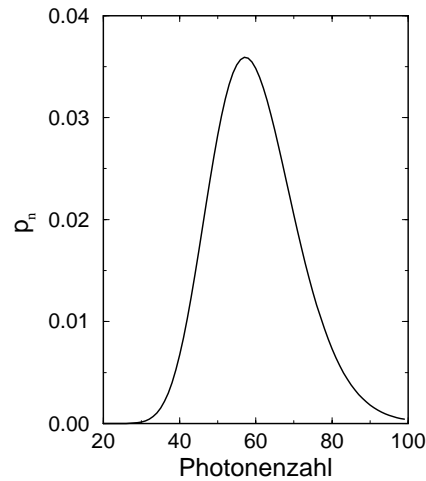
Abbildung 4.6: Photonenstatistik eines phasengequetschten Zustands der mittleren Photonenzahl \langle n \rangle = 60 und dem Quetschparameter \xi = 0,7i .
