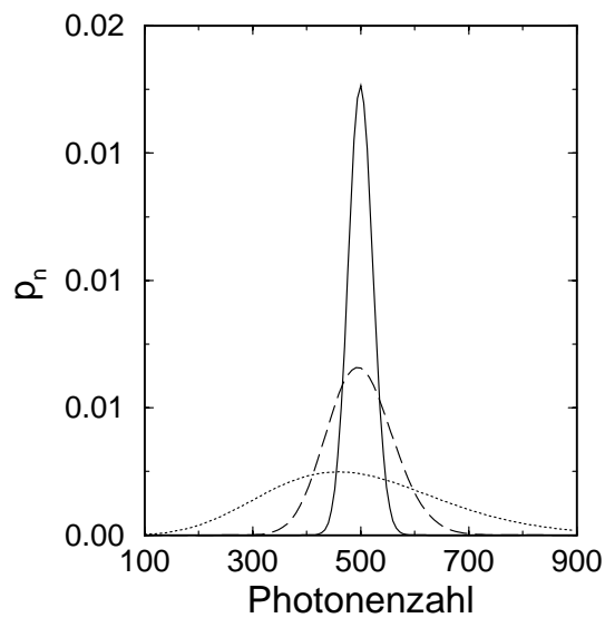
Abbildung 4.9: Photonenzahlstatistik der in Abb. 4.8 angenommenen Pumpfelder. Durchgezogene Kurve: \xi = 0 , gestrichelte Kurve: \xi = 1 , gepunktete Kurve: \xi = 2 .
