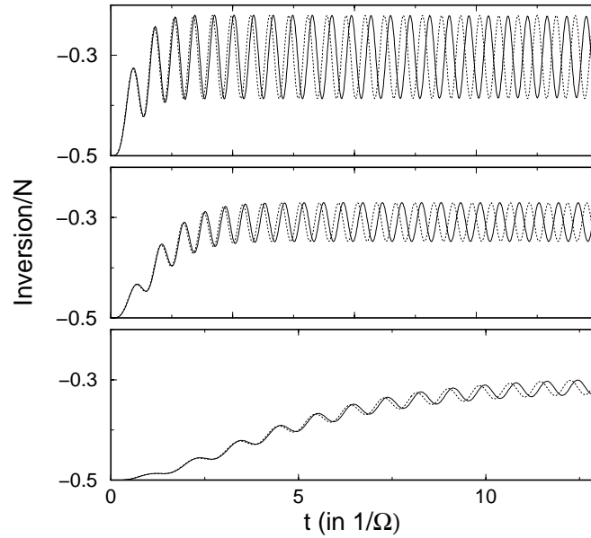
Abbildung 4.17: Vergleich der exakten (durchgezogene Kurven) und genäher- ten (gepunktete Kurven) Zeitentwicklung der Inversion für unterschiedliche Ein- schaltzeiten \tau_p . Das Pumpfeld ist im Fockzustand mit 60 Photonen. Oberes Bild: \tau_p \cdot \Omega = 1,6 , mittleres Bild: \tau_p \cdot \Omega = 3,2 , unteres Bild: \tau_p \cdot \Omega = 7,8 .
