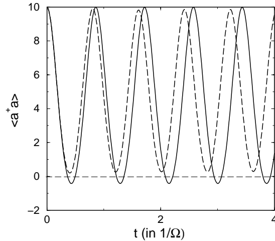
Abbildung 3.9: Zeitentwicklung der Pumpphotonenzahl in DMN (durchgezogene Kurve) und in EDMN (gestrichelte Kurve) für ein Pumpfeld im Fockzustand. In der DMN treten unphysikalische negative Werte auf. Parameter: N = 20 , n = 10 , \Delta = 0,6g .
