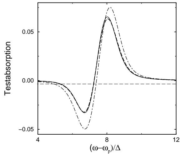
Abbildung 3.13: Testabsorption mit den Parametern aus Abb. 3.10; durchgezogene Kurve: exakt, strichpunktierte Kurve: EDMN mit Standardentkopplung (3.31), gestrichelte Kurve: EDMN mit anregungszahlerhaltender Entkopplung (3.33).
