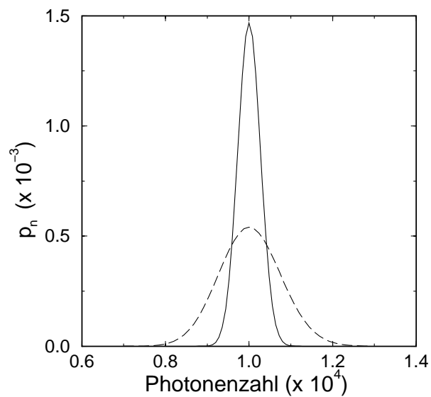
Abbildung 4.11: Photonenzustand der in Abb. 4.10 angenommenen Pumpfelder.
