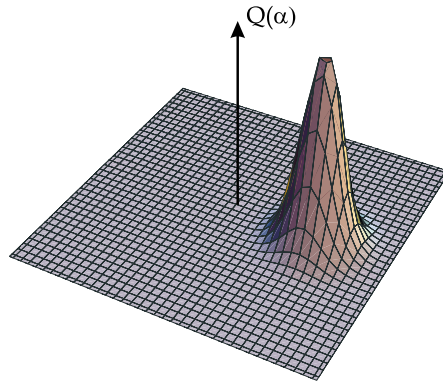
Abbildung 2.2: Q-Funktion eines kohärenten Feldes.
