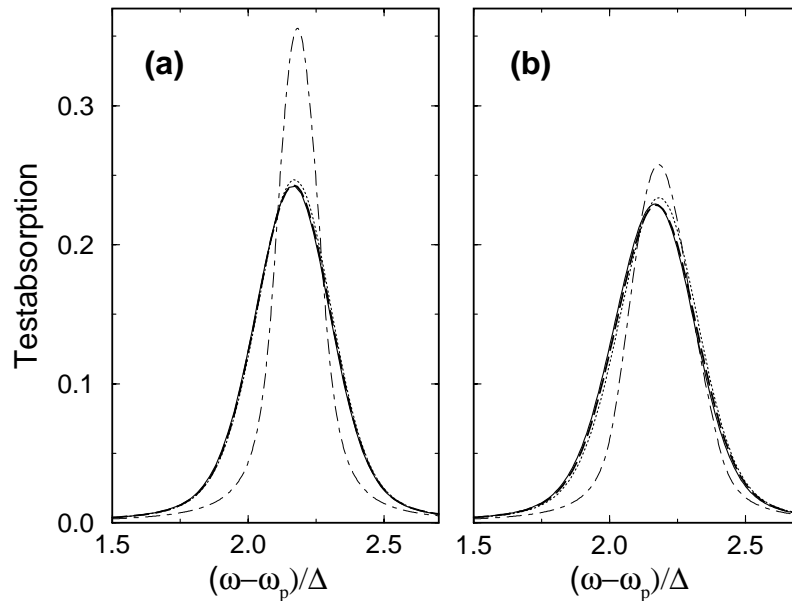
Abbildung 4.2: Testabsorption für ein kohärentes Pumpfeld für (a) \Gamma = 2g , (b) \Gamma = 3,2g . Durchgezogene Kurve: exakt; gepunktete Kurve: DMN mit Standardentkopplung gemäß (3.11); gestrichelte Kurve: DMN mit anregungszahlerhaltender Entkopplung (4.19). Parameter: N = 5 , \langle n \rangle = 60 , \Delta = 8g , \gamma = 0,4g . Die dünnen strichpunktierten Kurven zeigen die semiklassischen Testabsorptionsspektren mit inhomogener Verbreiterung.
