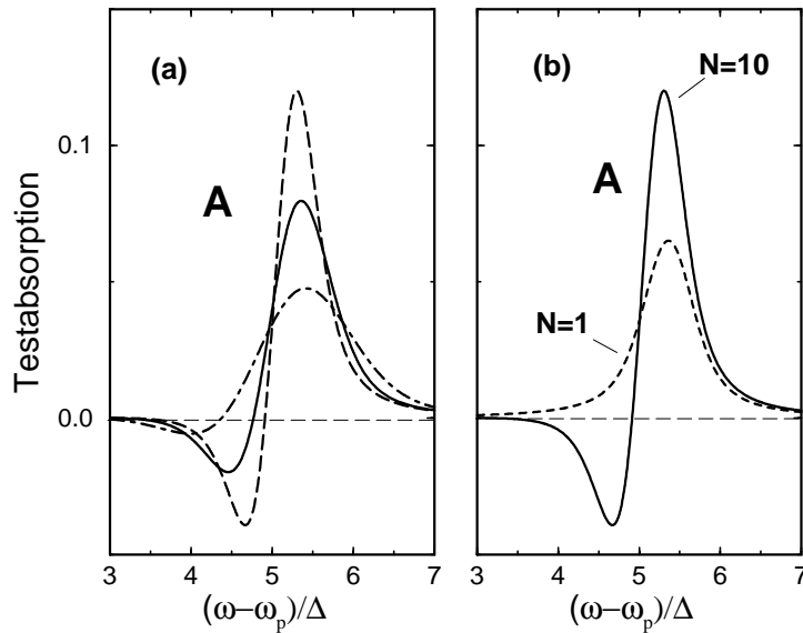
Abbildung 2.16: (a) Testabsorption mit nichtklassischer Verstärkung für zehn TLS und unterschiedlich gequetschte Pumpfelder. Gestrichelte Kurve: \xi = 0,5 ; durchgezogene Kurve: \xi = 0 ; strichpunktierte Kurve: \xi = -0,5 . (b) Testabsorption für zwei unterschiedliche Zahlen N von TLS für \xi = 0,5 . Weitere Parameter: \Delta = 3g , \langle n \rangle = 60 , \gamma = 0,8g .
