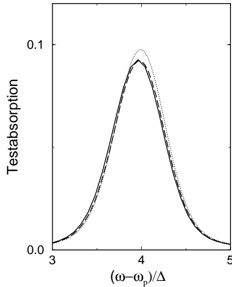
Abbildung 4.3: Testabsorption für ein kohärentes Pumpfeld mit inhomogener Verbreiterung \Gamma = 2g . Durchgezogene Kurve: exakt; gepunktete Kurve: DMN mit Standardentkopplung (3.11); gestrichelte Kurve: DMN mit anregungszahlerhaltender Entkopplung (4.19). Parameter: N = 5 , \langle n \rangle = 60 , \Delta = 4g , \gamma = 0,4g .
