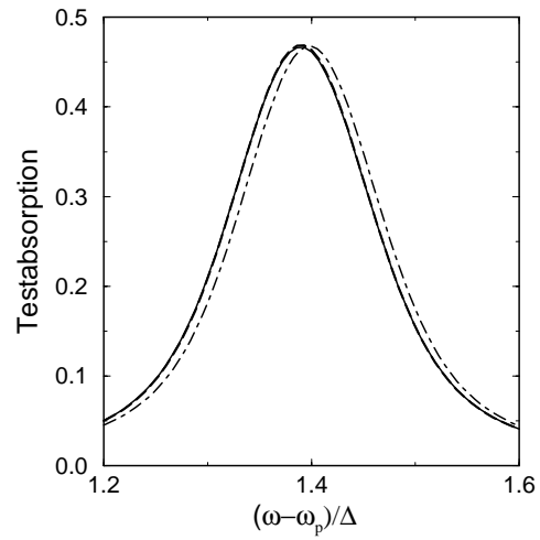
Abbildung 3.12: Testabsorption für ein kohärentes Pumpfeld mit den Parametern aus Abb. 3.4. Durchgezogene Kurve: exakt; gestrichelte Kurve: EDMN; strichpunktierte Kurve: DMN.
