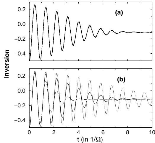
Abbildung 3.1: (a) Zeitentwicklung der Inversion in DMN für ein kohärentes Pumpfeld (gestrichelte Kurve) im Vergleich mit der exakten Zeitentwicklung (durchgezogene Kurve) für N = 10 . (b) Zeitentwicklung der Inversion in DMN für unterschiedlich gequetschte Pumpfelder. Durchgezogene Kurve: \xi = 0 ; gepunktete Kurve: \xi = 0,7 ; gestrichelte Kurve: \xi = -0,7 . Weitere Parameter: \Delta = 8g , \langle n \rangle = 60 .
