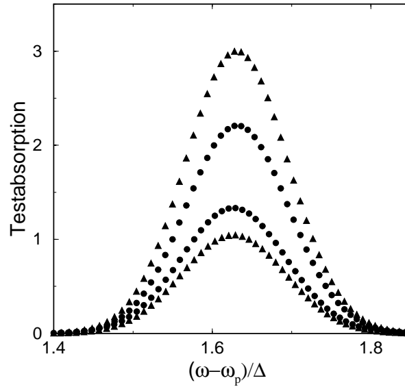
Abbildung 4.14: Testabsorption mit Unterstrukturen für N = 2 und zwei unterschiedliche Einschaltzeiten \tau_p . Kreise: \tau_p \cdot \Omega = 0,16 ; Dreiecke: \tau_p \cdot \Omega = 0,31 . Parameter: \Delta = 16g , \langle n \rangle = 60 , \xi = 0 .
