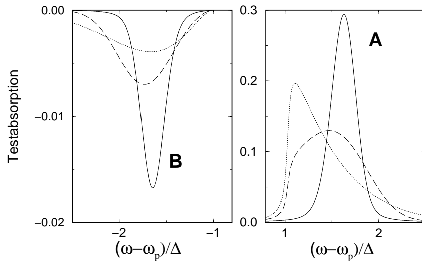
Abbildung 2.10: Testabsorptionsspektren für die Photonenzahlverteilung der Laseremission aus Abb. 2.9. Parameter: N = 1 , \Delta = 12g . Es ist eine homogene Verbreiterung von \gamma = 0,4g angenommen worden.
