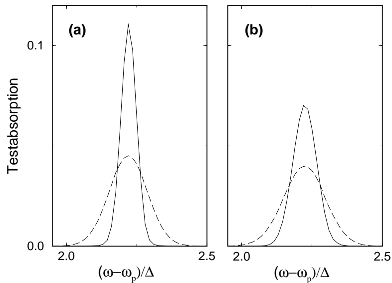
Abbildung 4.10: Testabsorption für 500 Störstellen. Das Pumpfeld ist in phasengequetschten Zuständen mit \langle n \rangle = 10^4 , deren jeweilige Photonenzustand in Abb. 4.11 gezeigt ist. Inhomogene Verbreiterungen: (a) \Gamma = 5g , (b) \Gamma = 15g . Weitere Parameter: \Delta = 100g , \gamma = 0,12g .
