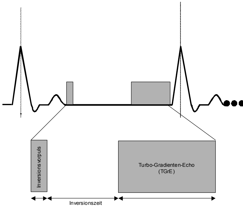
Abbildung 3: Pulssequenz zur Perfusionmessung. Auf den Inversionsvorpuls folgt die Datenakquisition in einer Schicht mit einer Turbo-Gradientenecho-Technik.
