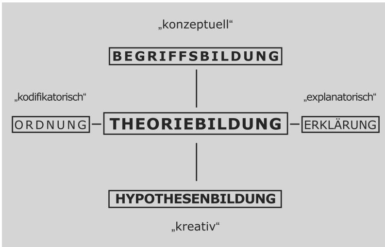
Abb. 4: Funktionen von Theorien
