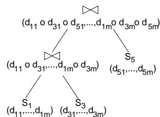
Abbildung 3: Ein Anfrageplan mit IQ-Vektoren und aggregierten IQ-Vektoren
