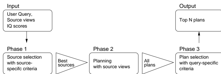
Abbildung 4: Drei-Phasen Anfrageplanung
