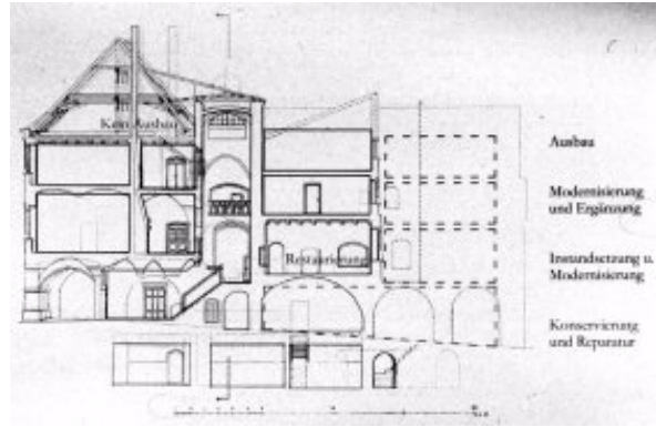
Abb.6: «Stufen» und «Themen» des Eingriffs in ein Denkmal. Konzeptzeichnung für die Umgestaltung des Hauses Untermarkt 25 in Görlitz. Diplomarbeit Maja Polenz, TU Dresden, Lehrstuhl für Denkmalpflege und Entwerfen, Sommer 2003.
